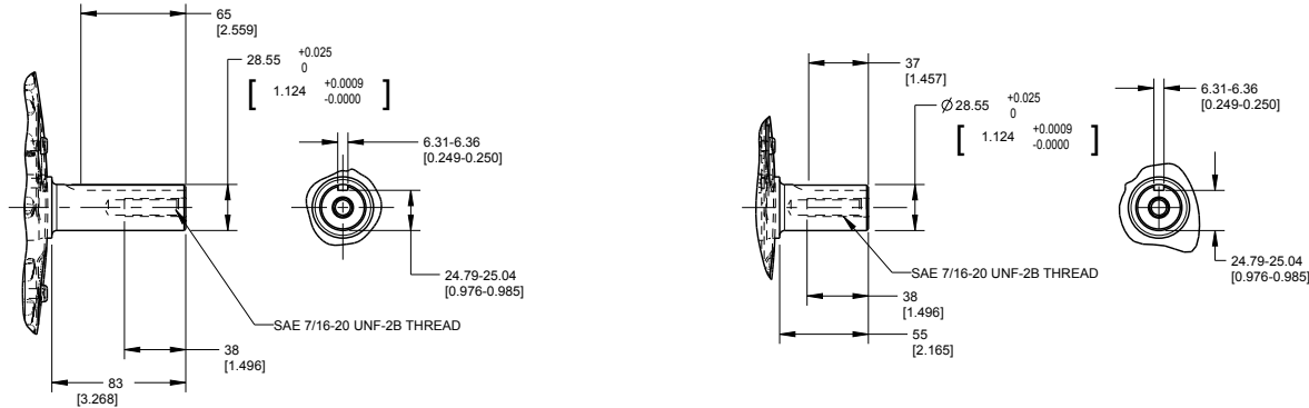
OPTIONAL LONG FRONT P.T.O.
